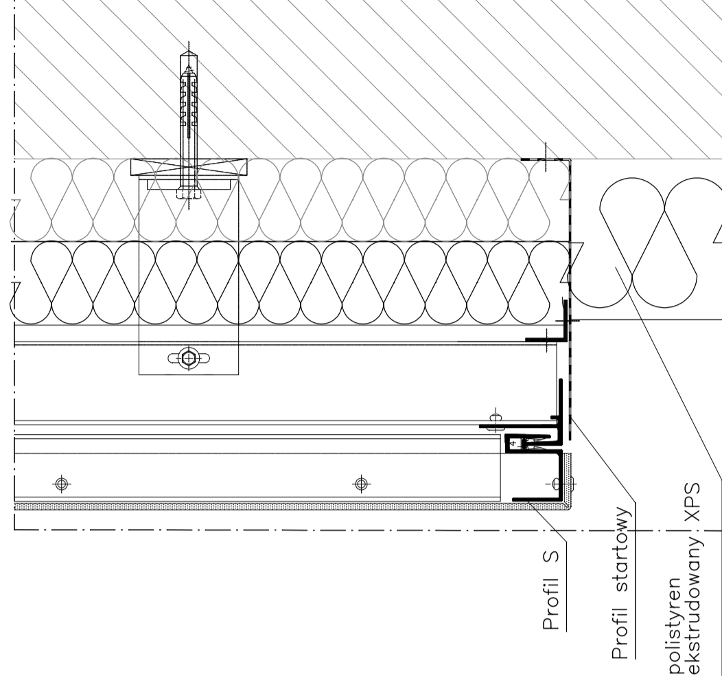
Detail cokołu
