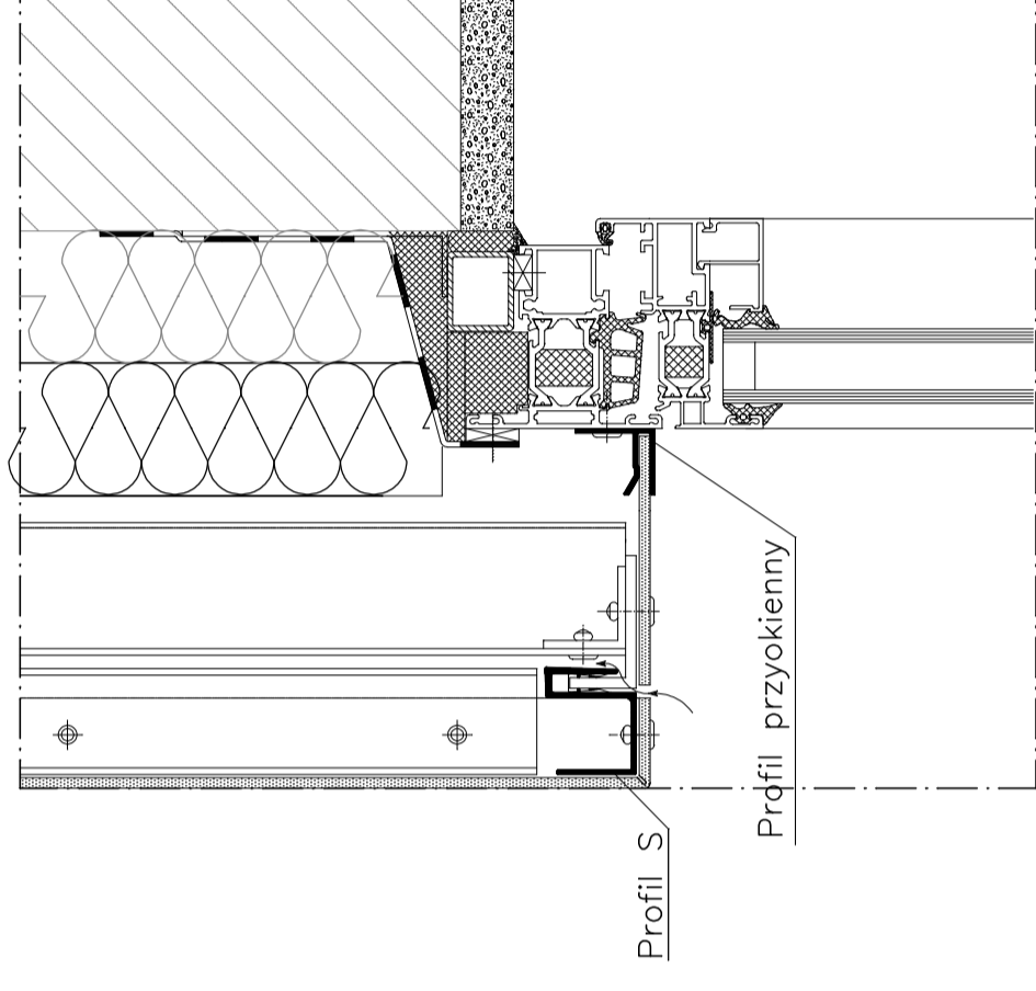
Detail połączenia z oknem
