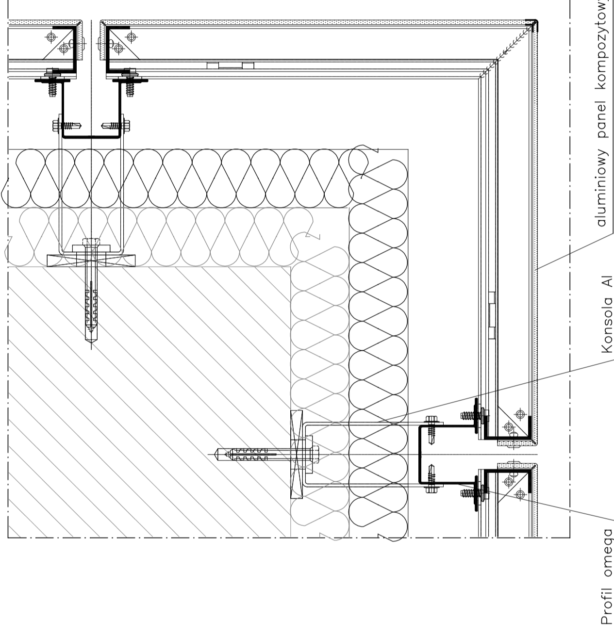
Detail naroża
